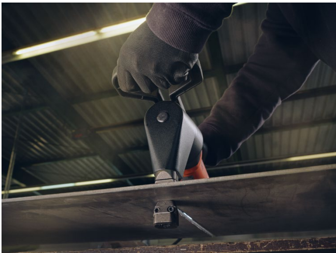
Imagen: La nueva BLK 5.0 E sigue siendo adaptable y versátil incluso en el corte de chapas metálicas de hasta 5 mm de grosor y proporciona un mecanizado sin chispas.
