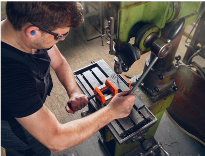
Imagen: el 30% de premagnetización permite alinear el tornillo de banco magnético de forma precisa.
