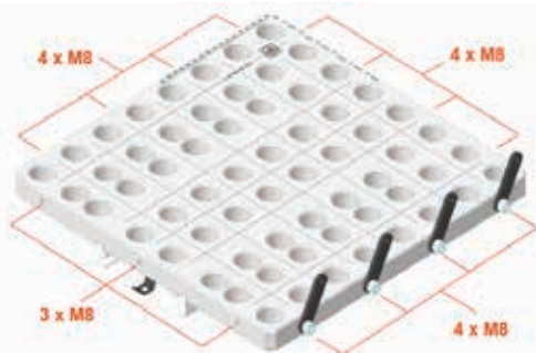
Svařovací deska s vnitřním závitem M8
