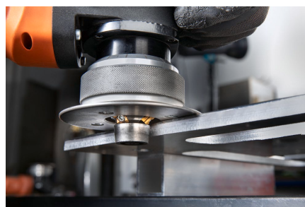
Bildunterschrift: Präzises Fräsen von Fasen – hier im Bild: die FEIN Akku-Kantenfräse AKFH 18-5 mit SX-Wendeschnidplatten.
