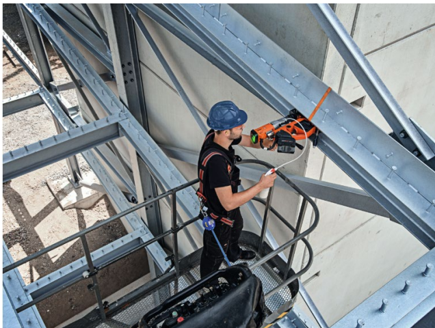
Bildunterschrift: Die AKBU 35 PMQW AS ist die einzige Akkukernbohrmaschine im AMPShare 18V Akkusystem.
