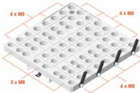
Zvárací doska s vnútorným závitom M8
